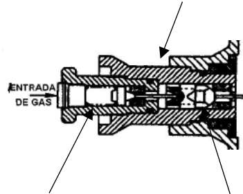
Válvula de seguridad primaria
